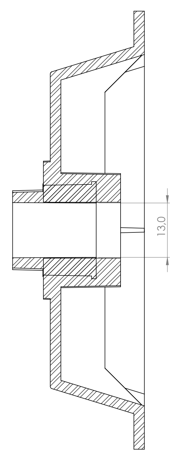
SEÇÃO B-B
