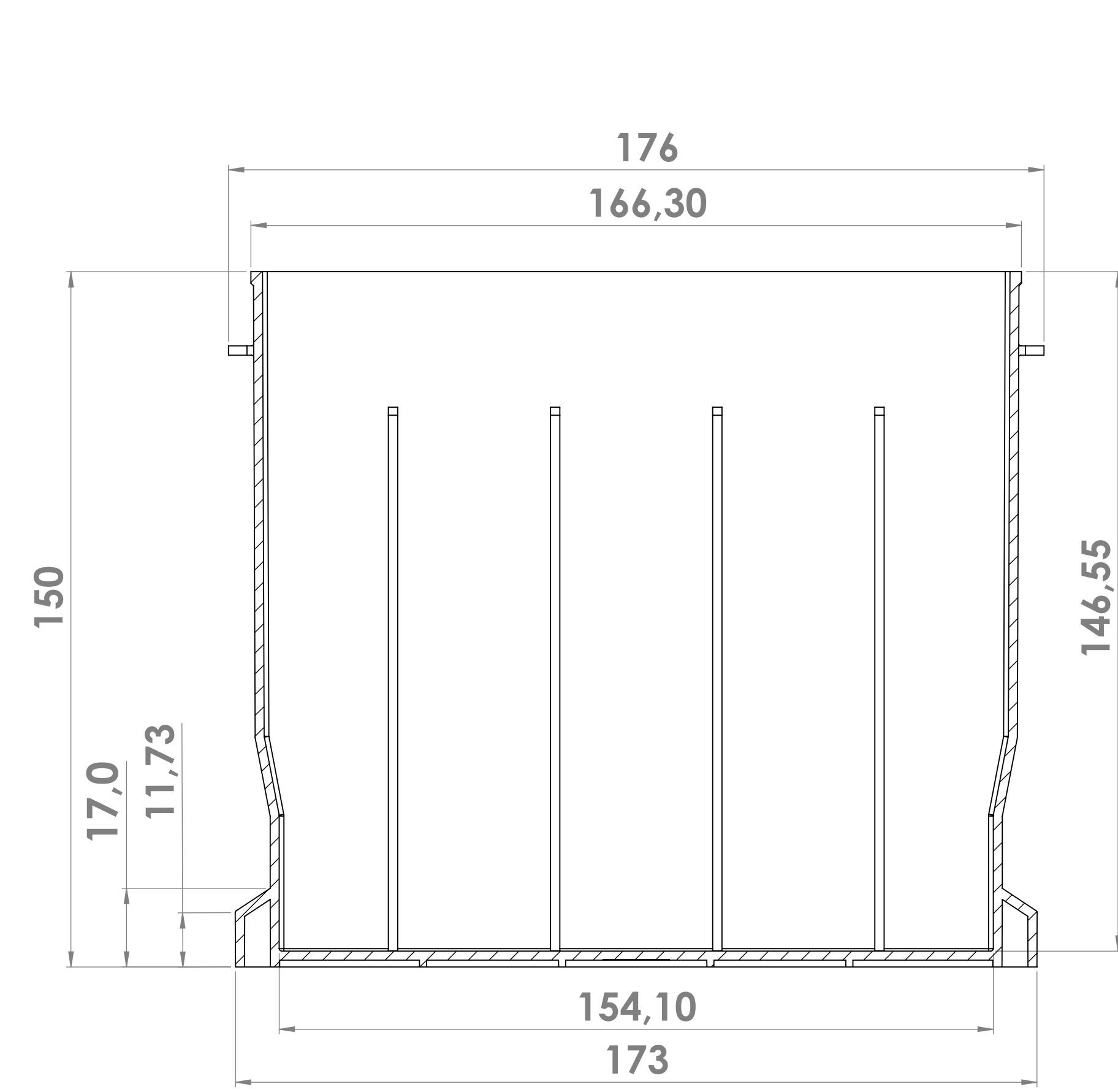
SEÇÃO A-A
